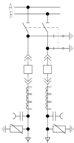
Ячейка КРУ двухфазного фидера ДПР
