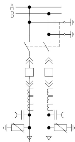
Ячейка КРУ двухфазного ввода
