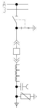
Ячейка КРУ фидера КС
