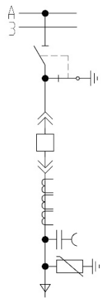
Ячейка КРУ фидера ЗВ
