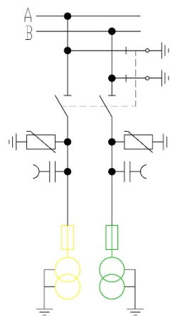
Ячейка КРУ двухфазного трансформатора напряжения
