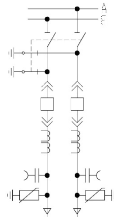
Ячейка КРУ двухфазного фидера ТСН
