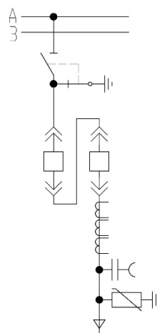
Ячейка КРУ фидера УК
